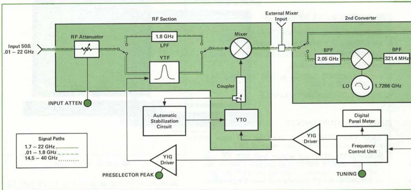
Figure 44. HP 8565A block di.
